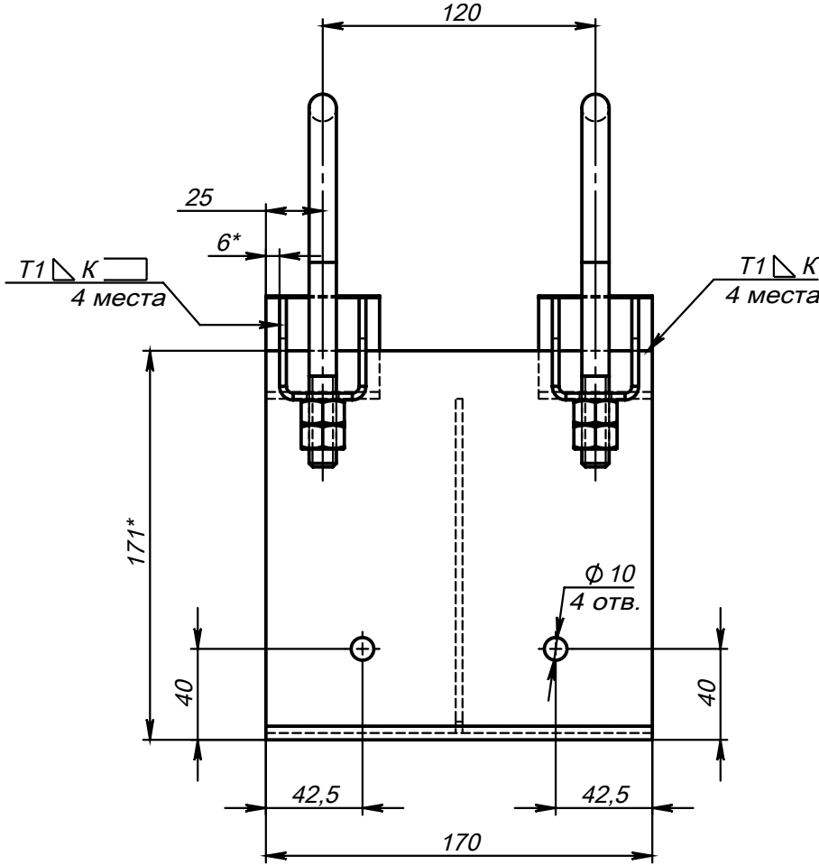
Поз.4 (Ложement)
