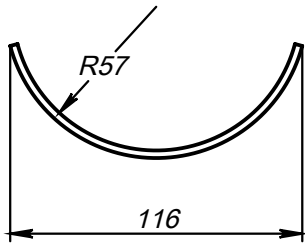
Поз.3 (Хомут)
